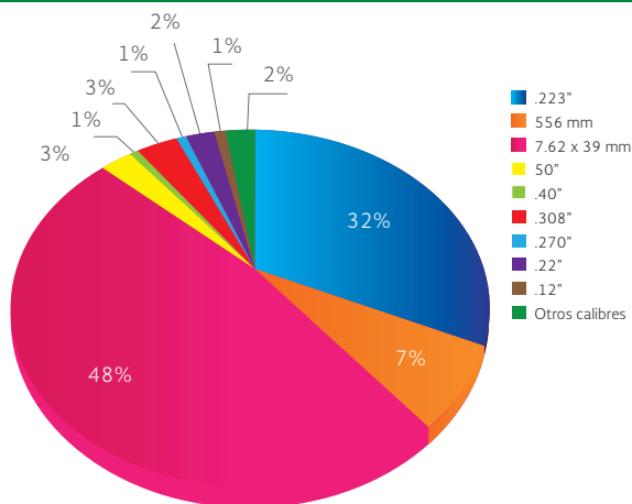
Gráfica 3. Aseguramiento de armas de fuego largas por calibre. 1 de septiembre de 2015 a 30 de junio de 2016
